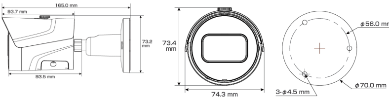
寸法図 (mm)
