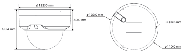
寸法図 (mm)
